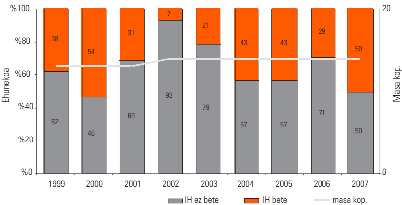
II.3.7. GRAFIKOA. TRANTSIZIOKO UR-MASAK. MAKROORNOGABEEN EGOERAREN BILAKAERA. M-AMBI INDIZEA
